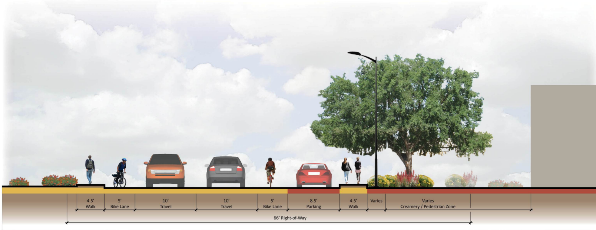
SECTION 3A - 3B
